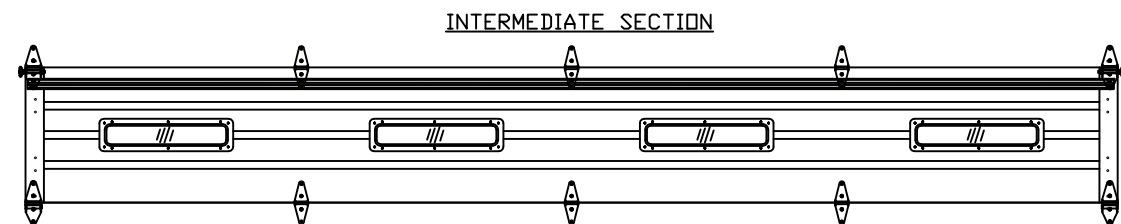
OPTIONAL GLAZED SECTION W/ 24" X 6" WINDOWS N.T.S.
