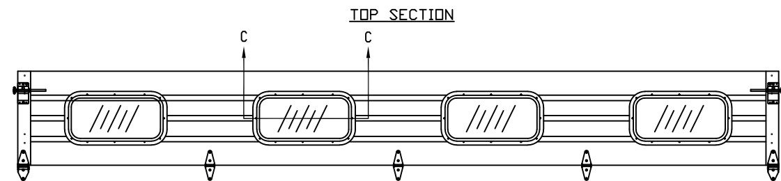
OPTIONAL GLAZED SECTION W/ 26" X 13" WINDOWS N.T.S.
